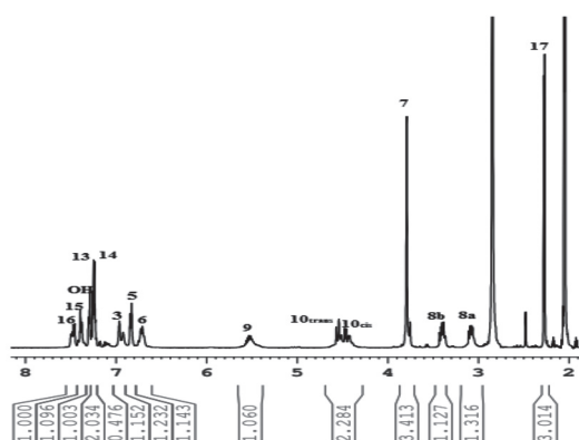
Hình 5a. Phổ ^1\text{H} NMR của phức [(\text{PtCl}_2(\text{Eug})(o\text{-toluidin}))]
