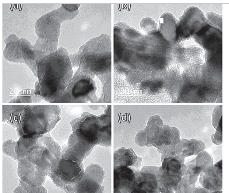
Hình 1. Ảnh TEM của bột TiN nguồn (a) và bột TiN được ủ trong không khí trong 2 giờ ở các nhiệt độ khác nhau: 300^\circ\text{C} (b), 350^\circ\text{C} (c) và 400^\circ\text{C} (d).
