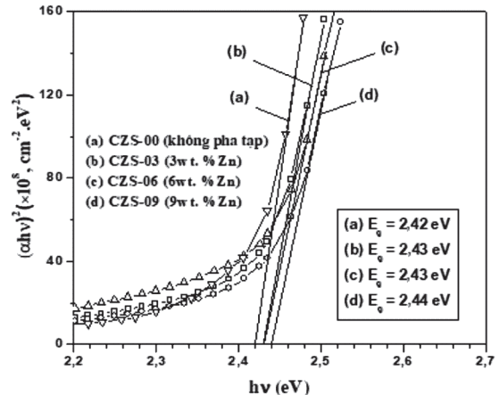
Hình 4. Đồ thị quan hệ (\alpha h\nu)^2 với h\nu của các mẫu CdS không pha tạp và CdS:Zn khảo sát
